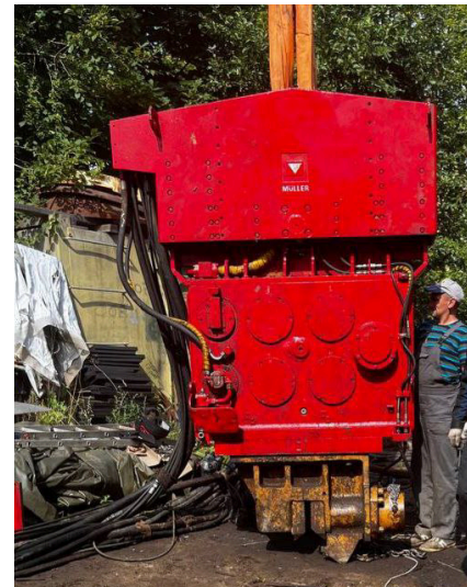
Вибропогрузатель MULLER MS-16HFV
